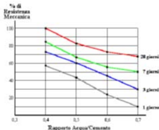
Fig. 1 – Diagramma resistenza meccanica c.a. - rapporto acqua/cemento
