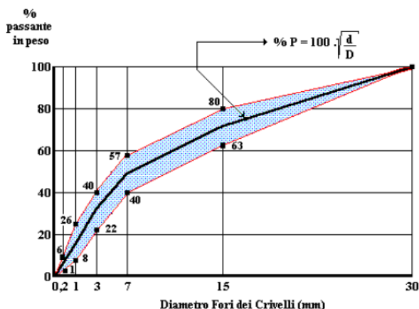
Fig. 2 – Distribuzione granulometrica degli inerti – curva teorica di Fuller
