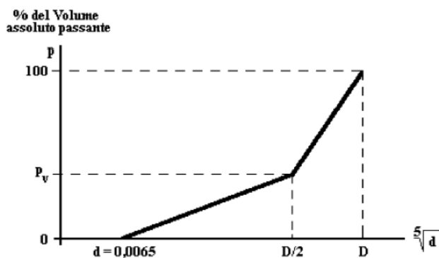
Fig. 3 – Distribuzione granulometrica inerti secondo la rappresentazione di Faury
